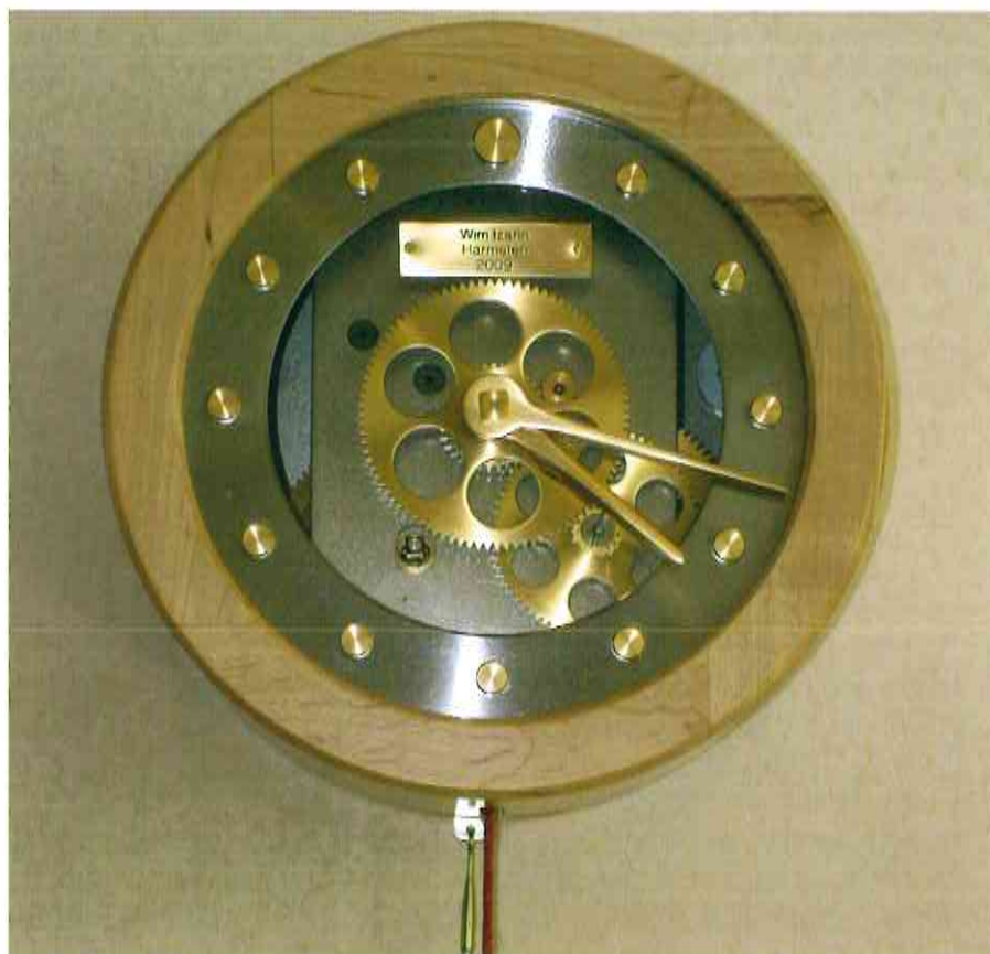
Afb. 1 - Doorkijk in het uurwerk
